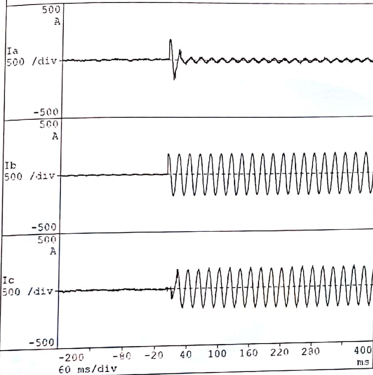
试验波形示波图
