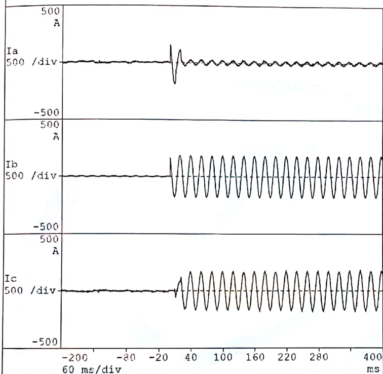
试验波形示波图
