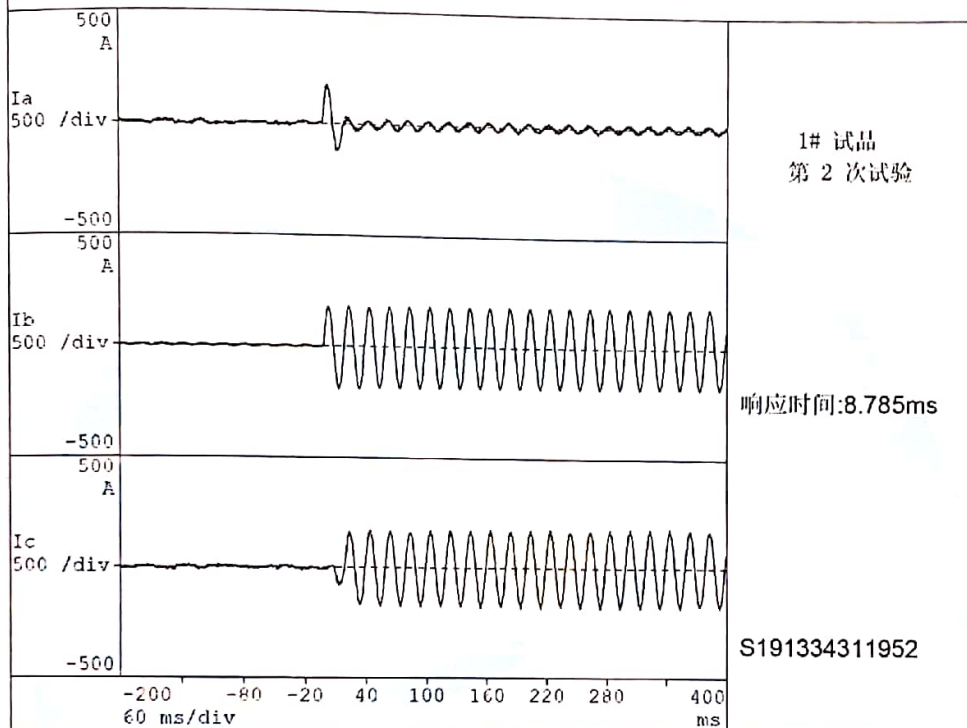
试验波形示波图
