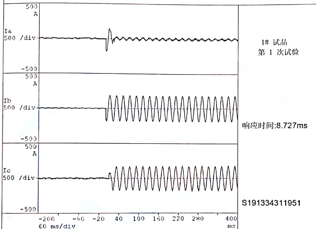
试验波形示波图
