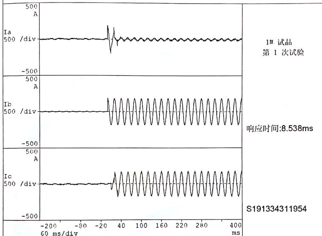
试验波形示波图
