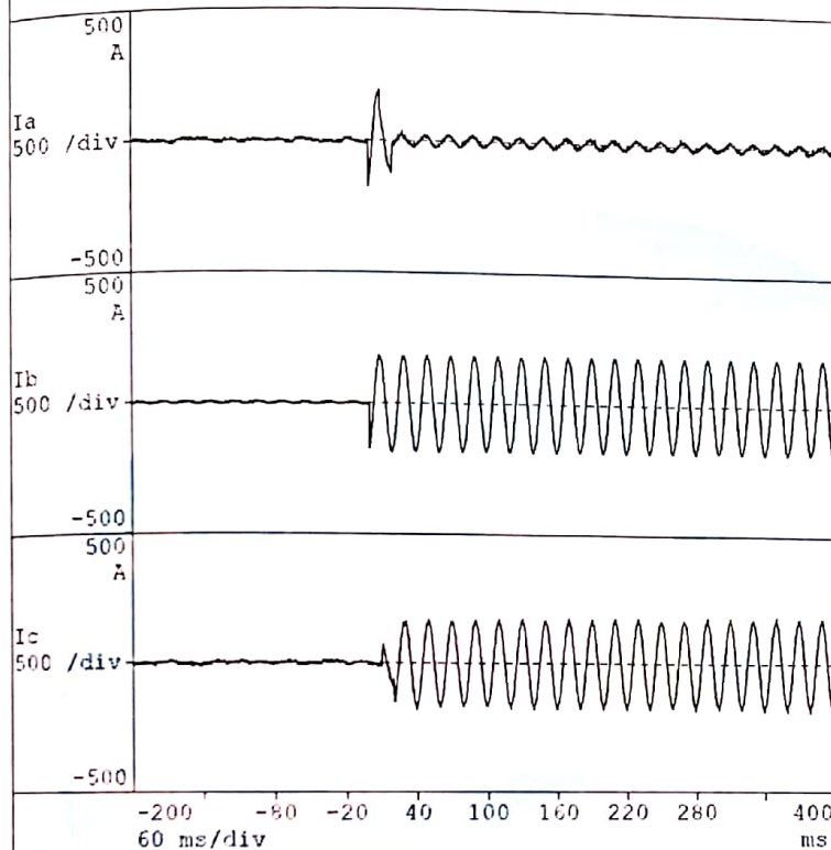
试验波形示波图
